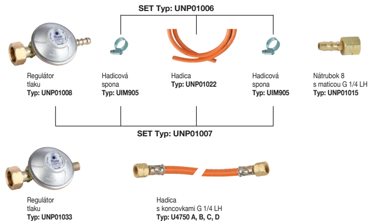
nízkotlakový varič – pripojenie na 10 kg fľašu
